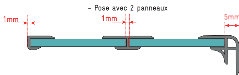
Profilé de jonction
