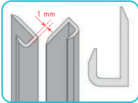
Abschlussprofil
