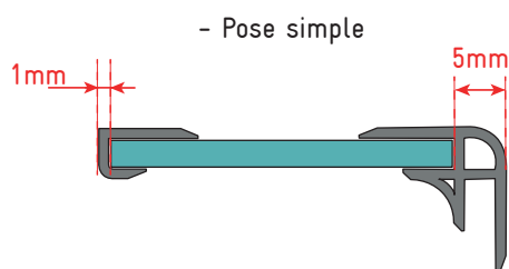
Profilé de finition
