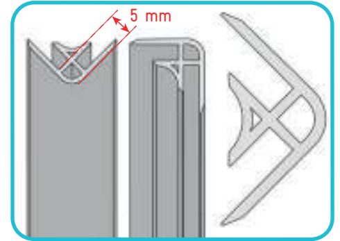
- Eckprofil
