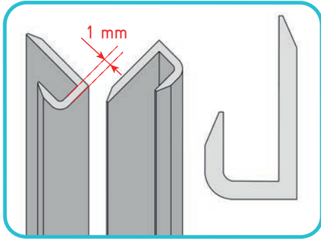
Abschlussprofil
