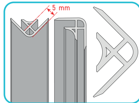
Profilo d'angolo
