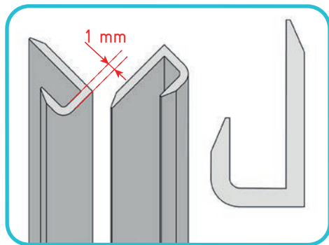
Edge profile
