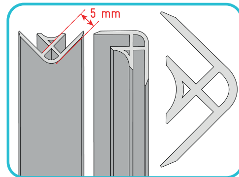
Profilo d'angolo
